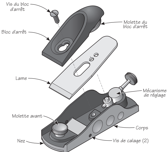
Figure 1 : Éléments du rabot
