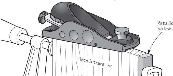
Figure 4 : Prévenir les éclats
