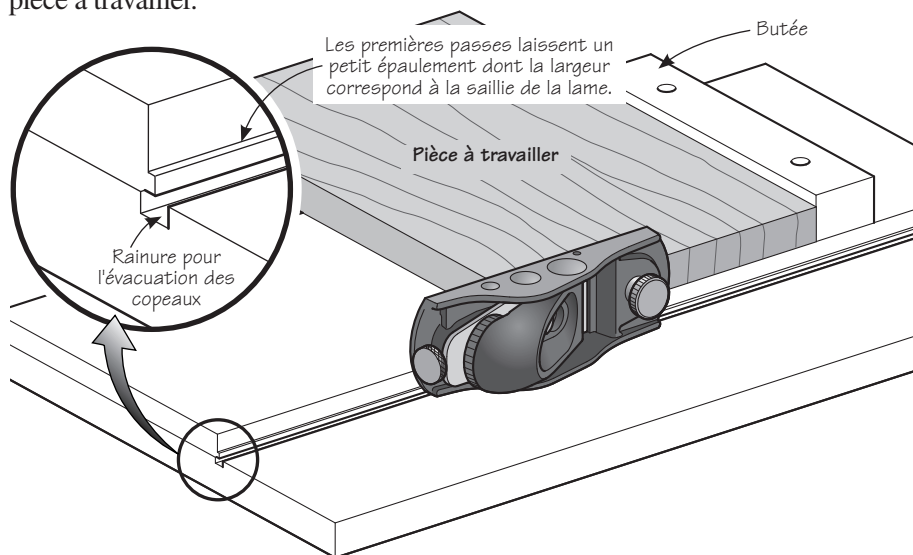
Figure 5 : Coupe de bois de bout à l'aide du rabot de coupe à angle faible
