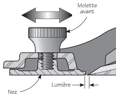
Figure 3 : Réglage de la lumière
